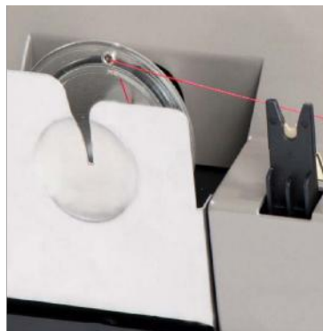
新型符合人体工学的热熔叉位置
